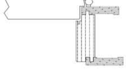
stipite alla trentina cornice standard
