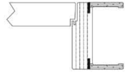
stipite standard con coprifilo a filo cerniere a scomparsa battuta easy
