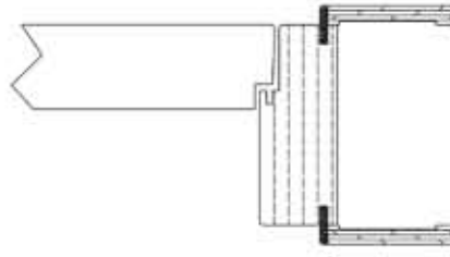
stipite standard con cerniere a scomparsa battuta easy
