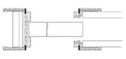
stipite standard per porta scorrevole interno muro
