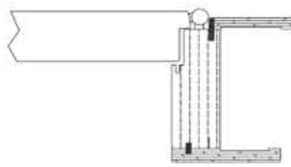
stipite a filo 90
