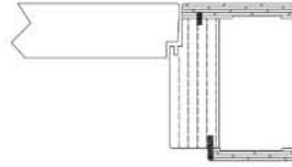
stipite filo interno cerniere a scomparsa battuta easy
