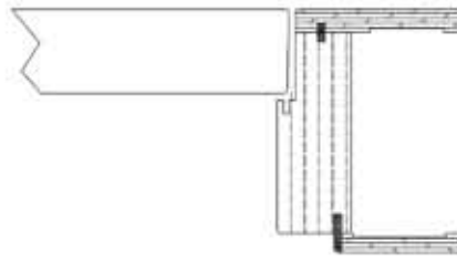
stipite a filo interno cerniere a scomparsa battuta standard
