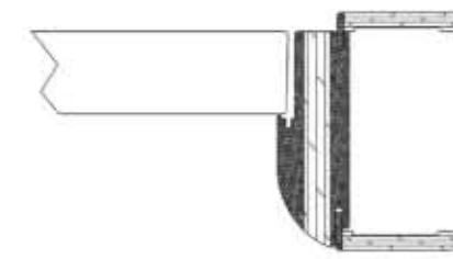
stipite raggio piano cerniere a scomparsa battuta standard
