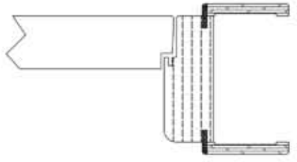
stipite R10 cerniere a scomparsa battuta easy
