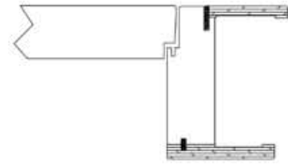
stipite a filo 90 cerniere a scomparsa battuta easy
