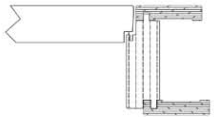
stipite alla trentina cerniere a scomparsa battuta easy
