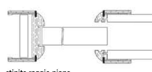
stipite raggio piano per porta scorrevole interno muro
