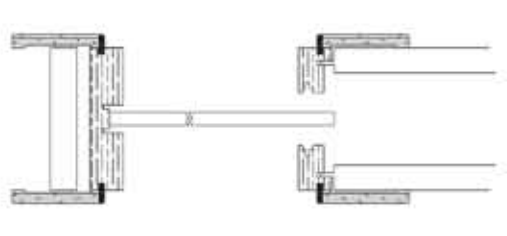
stipite standard per porta scorrevole interno muro tutto vetro
