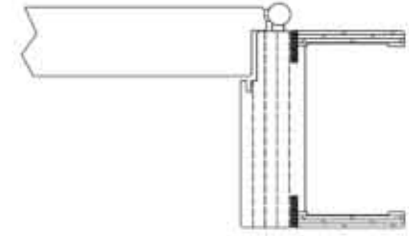
stipite standard con coprifili a filo cornice standard
