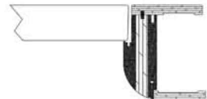
stipite raggio piano a filo interno cerniere a scomparsa
