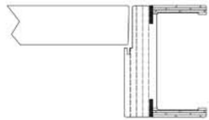
stipite standard con coprifilo a filo cerniere a scomparsa battuta standard
