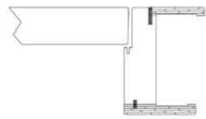
stipite a filo 90 cerniere a scomparsa battuta standard
