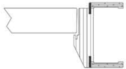
stipite prisma cerniere a scomparsa battuta standard
